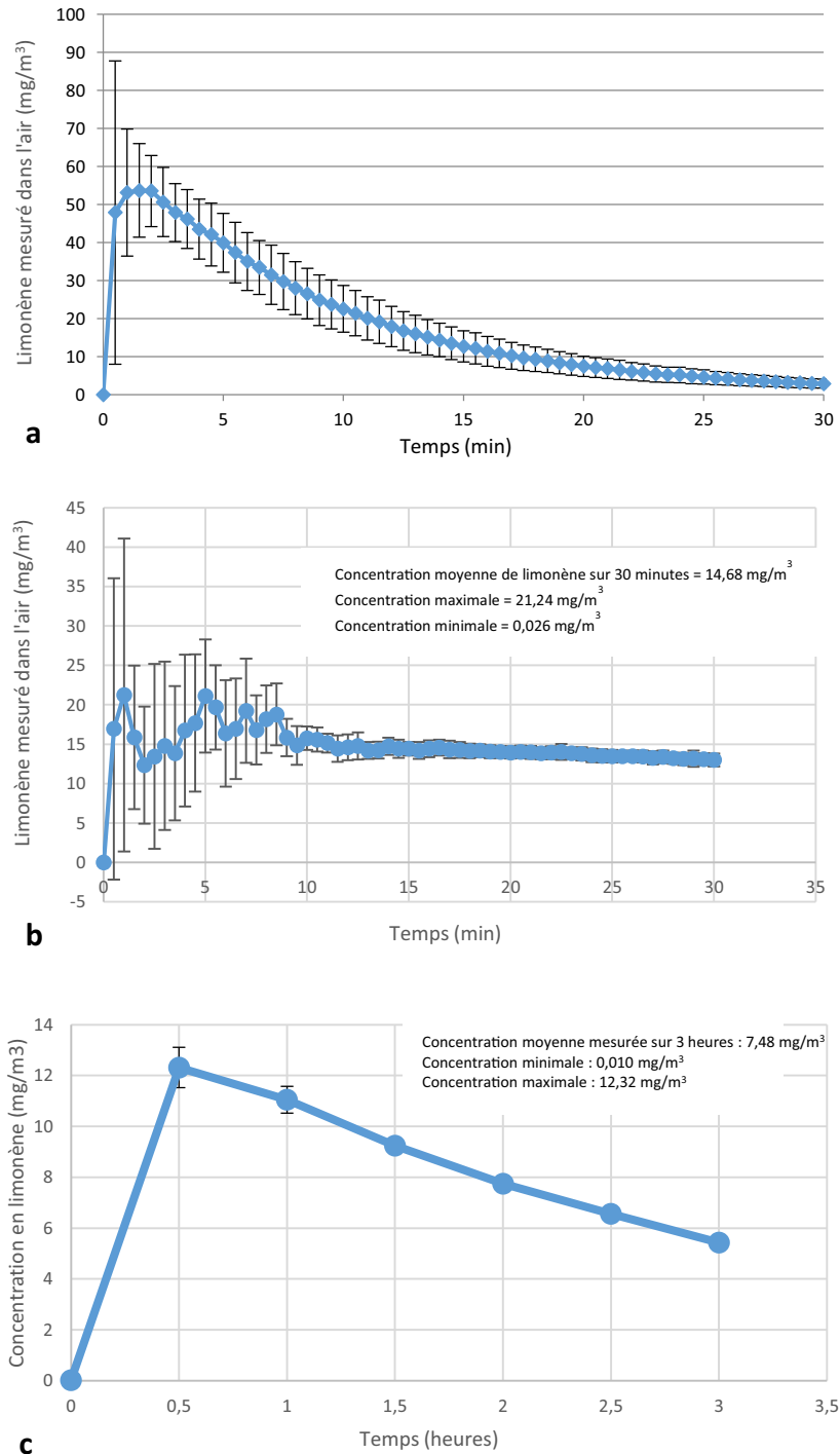
Fig. 1. Concentration moyenne de limonène mesurée dans l'air (mg/m 3 ) en fonction du temps (min) par méthode de photo-ionisation ; a : après 4 pulvérisations du spray aux 41 huiles essentielles ® dans une cabine de 9 m 3 ; b et c : après 8 pulvérisations du spray aux 41 huiles essentielles ® dans une pièce de 42 m 3 sur une période de 30 minutes et de 3 heures.
